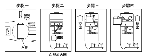
碳刷更换图
